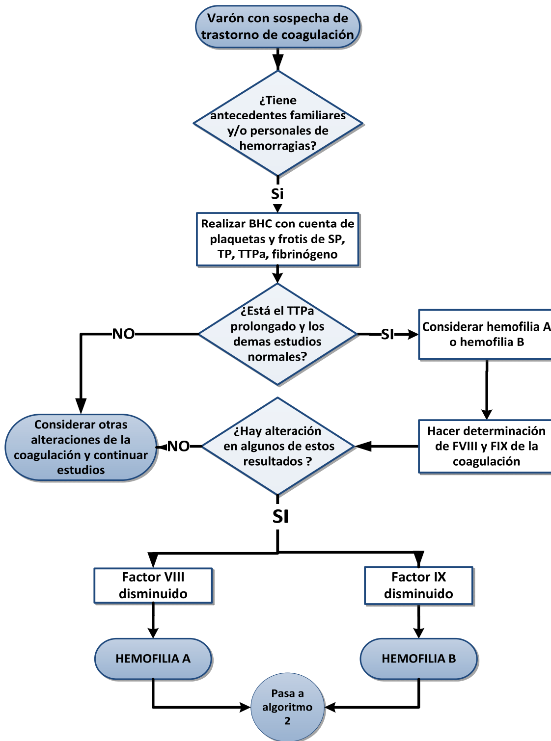
Algoritmo 1-Diagnóstico.
